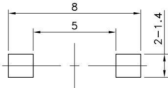
P.C.B TERMINAL POSITION
