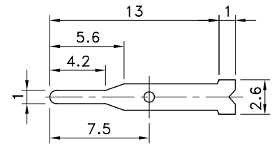
Terminal(C)
