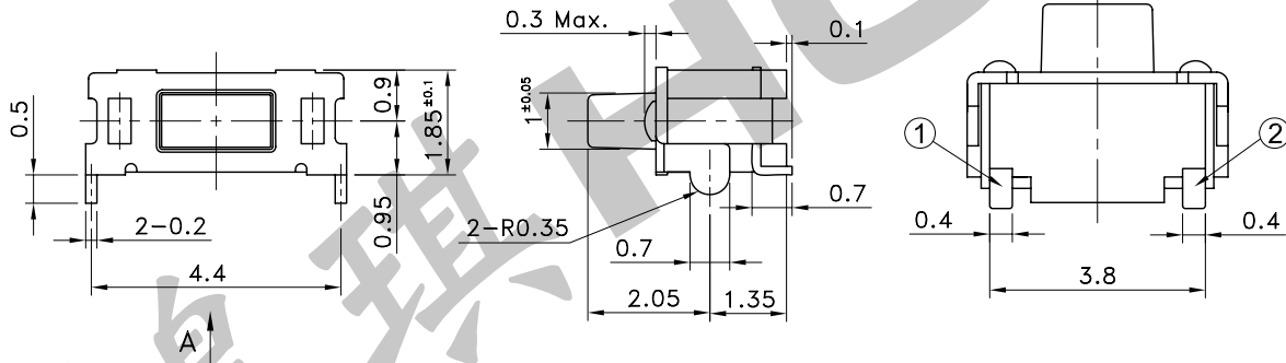
P.C.B TERMINAL POSITION
