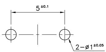
P.C.B TERMINAL POSITION
