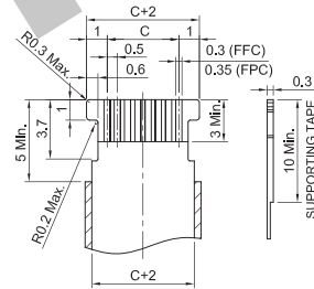
FPC • FFC Dimensions
